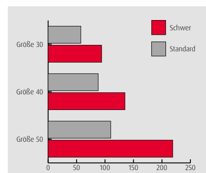
Abb. 2. Vergleich der statischen Tragzahl. Einheit: kN.
